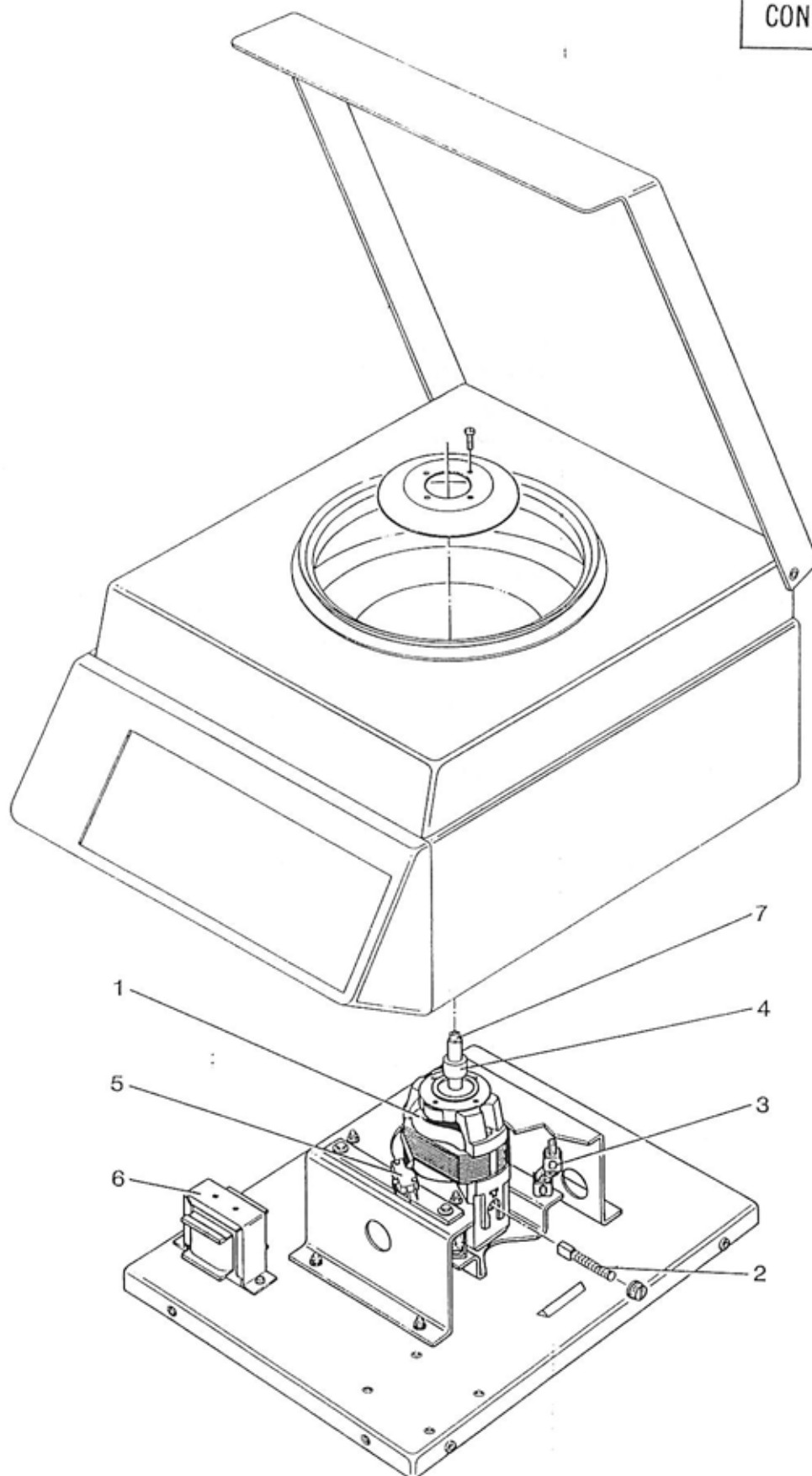
Figure 6.3 - MOTEUR MOTOR
