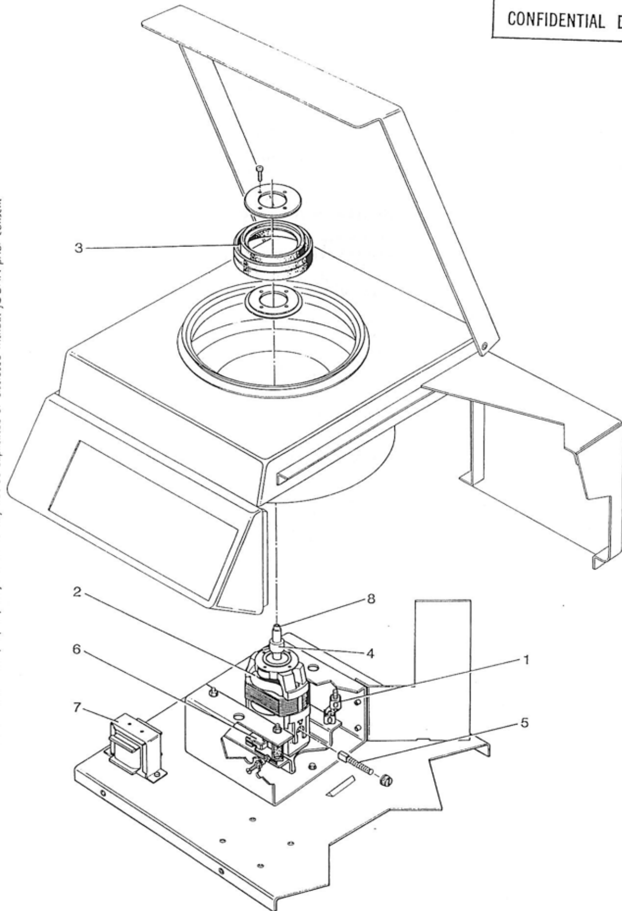
Figure 6.8 - MOTEUR MOTOR
