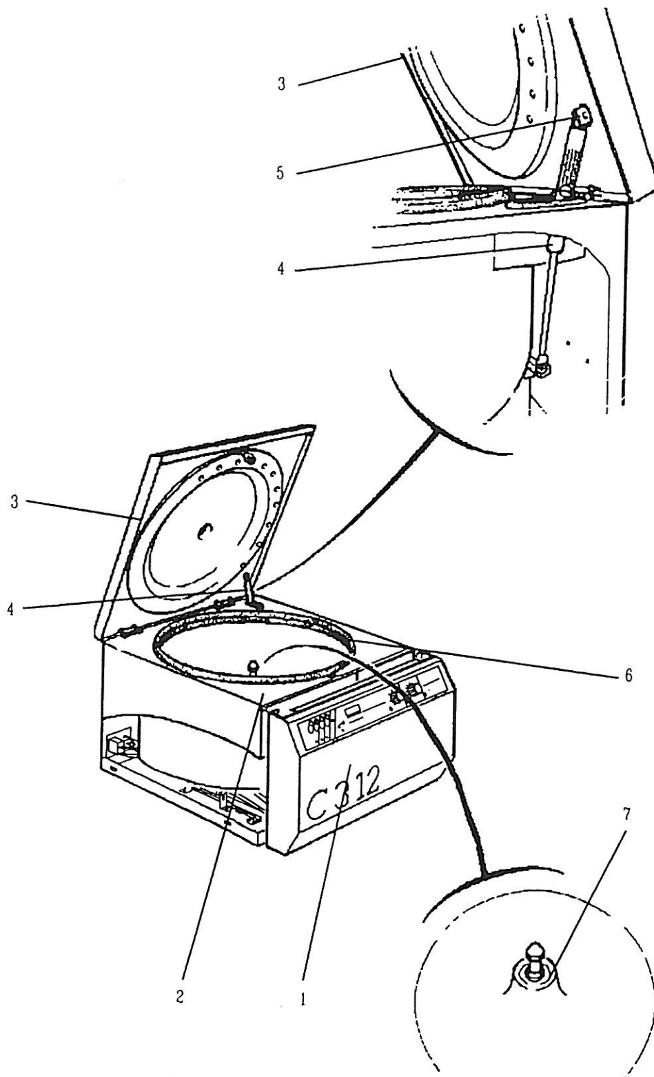
Figure 6.4.1 - VUE D'ENSEMBLE DU C3-12 GENERAL VIEW OF C3-12
